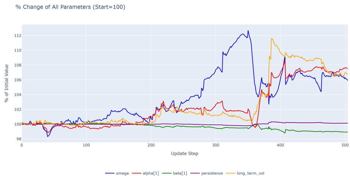
Figure 18: Parameter % Change over time
